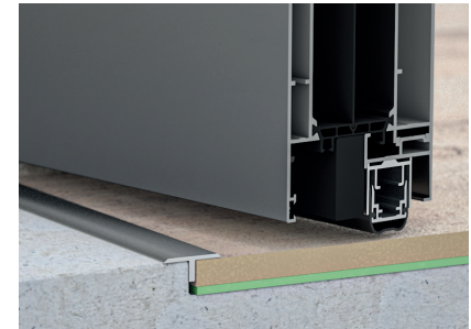
Schwelle mit automatischer Bodendichtung.
