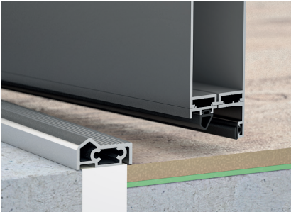
Schwelle mit Wölbung (standardmäßig).
